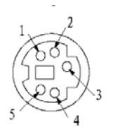
Mini Din 5 Pin Port
